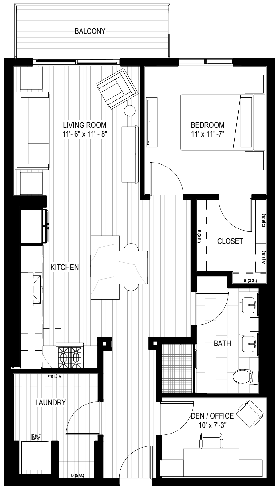
V-A1 900 SF
